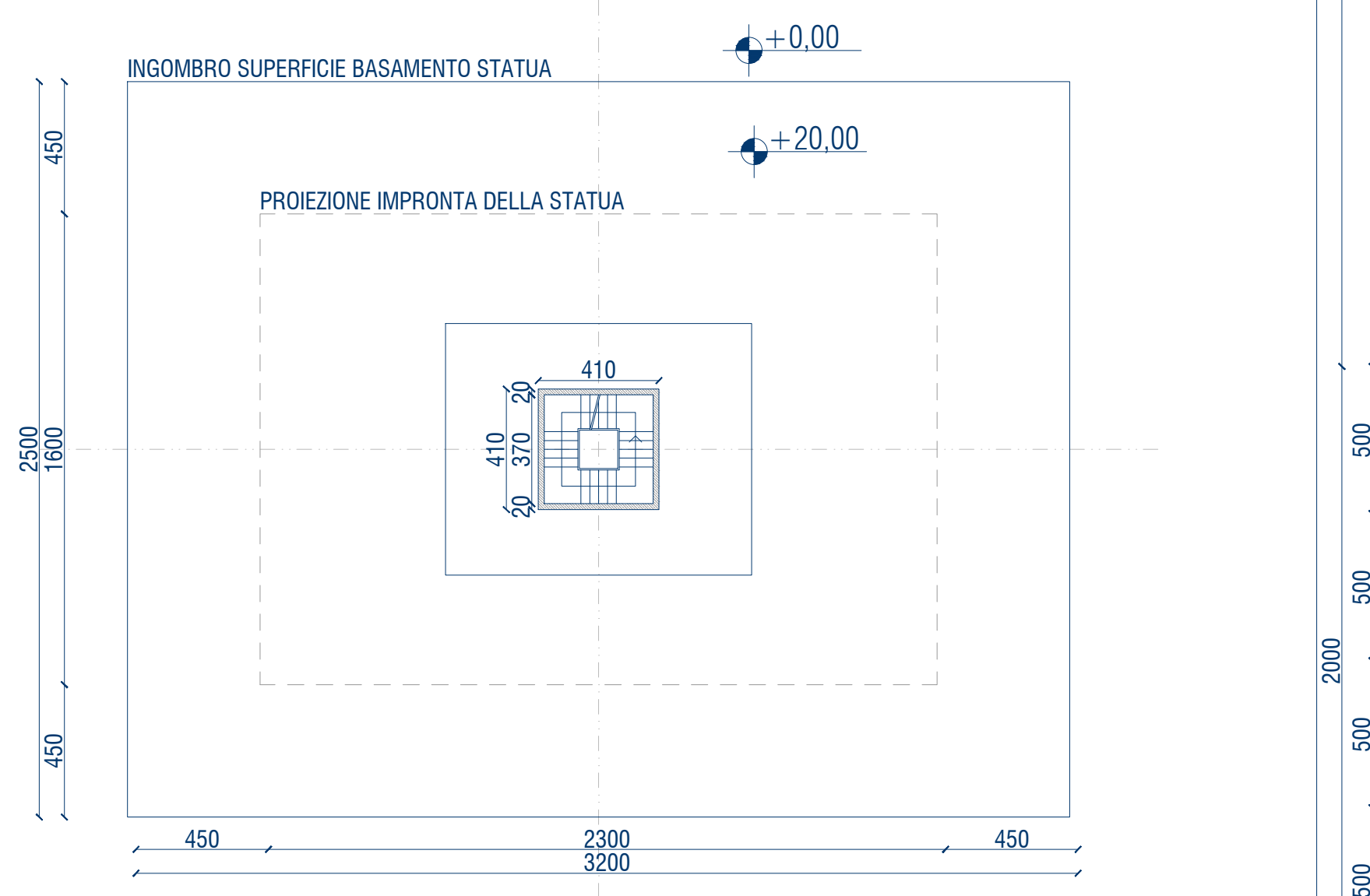
SEZIONE BB
